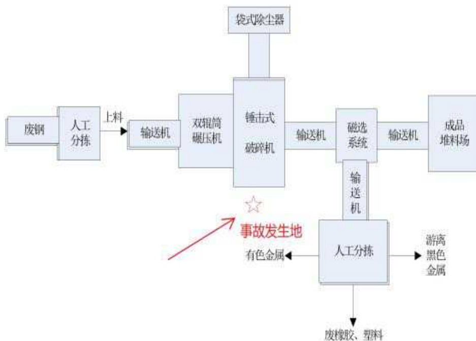
图 4 废钢破碎车间工艺流程图
