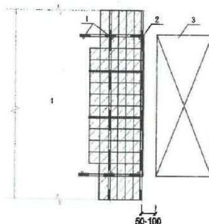
图 1：事故现场物料提升机与主体结构之间防护图片
