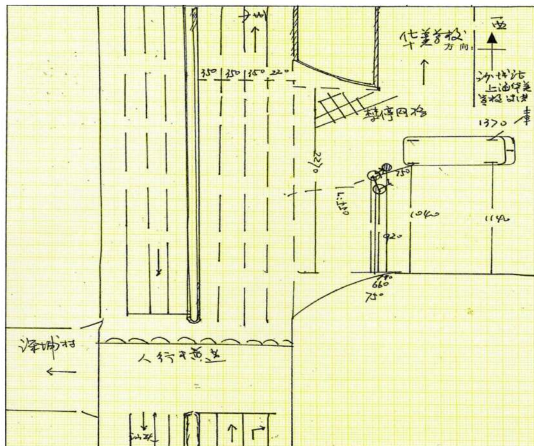
图 2 事故现场示意图
