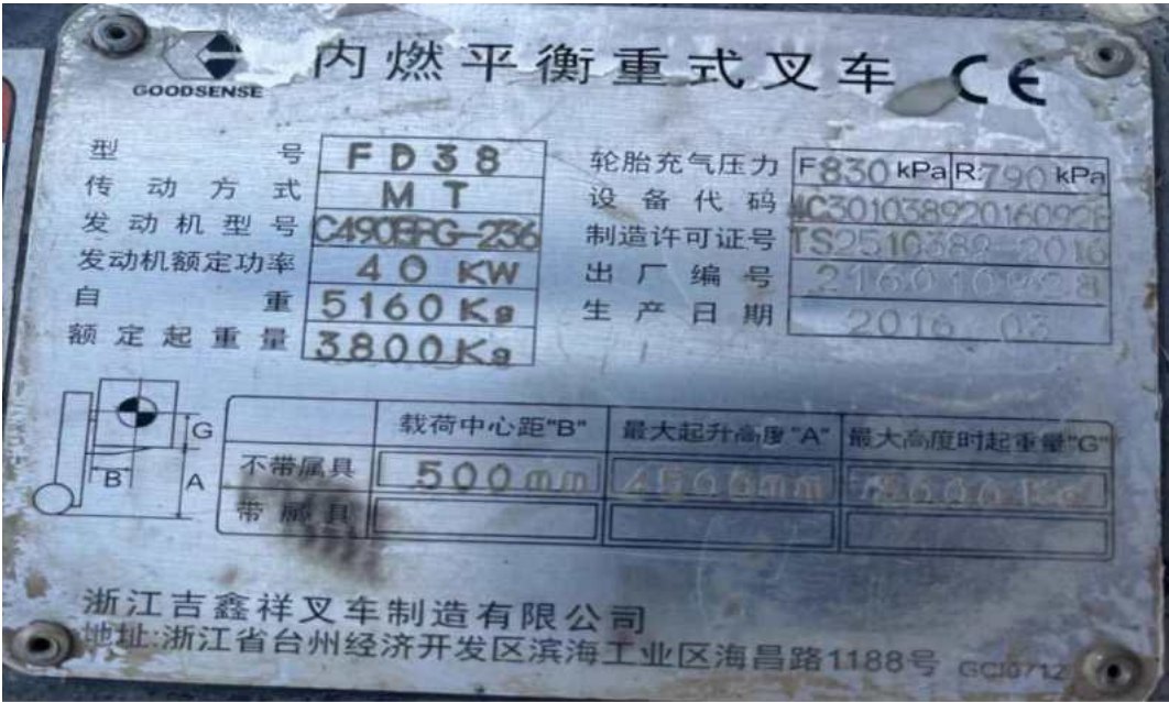
图片 1：内燃平衡重式叉车铭牌
