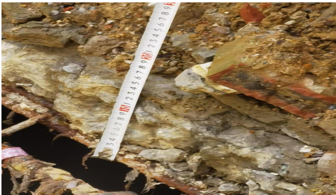
图 3. 现场勘查涵洞盖板情况
