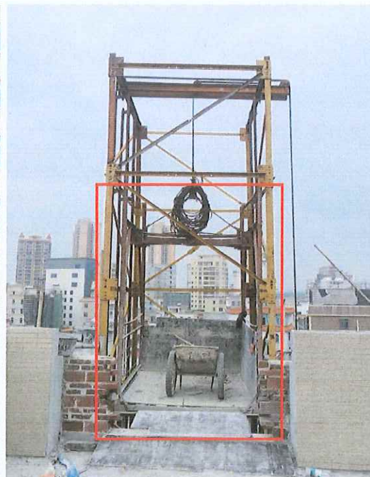
图 2 物料提升机吊篮
