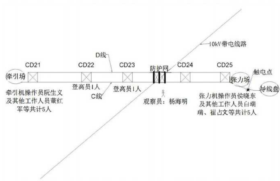
图 · 6月16日导线展放现场工作人员分布图
