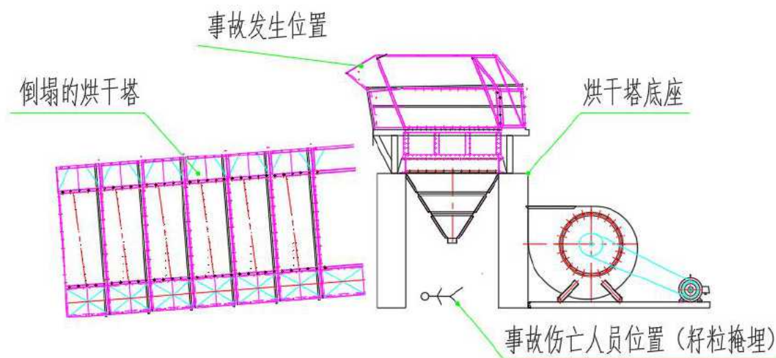
事故设备侧立面图
