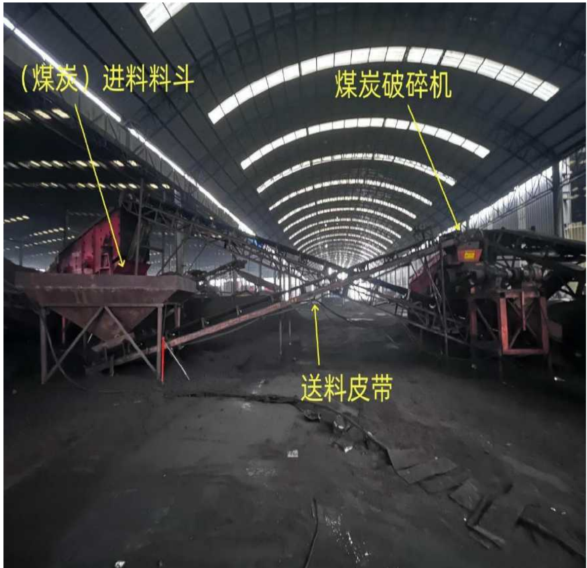
现场同类型机械图片
