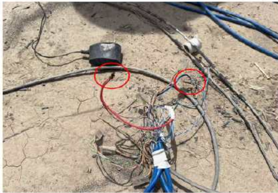
电源线线头裸露有烧灼痕迹
