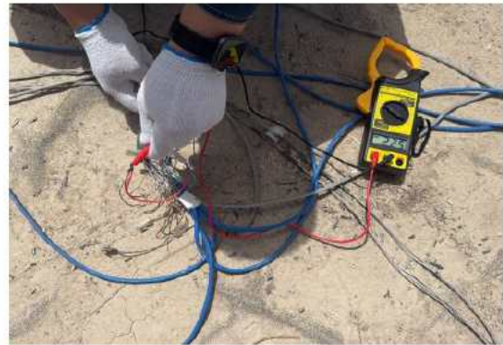
裸露零线-火线电压 225 伏
