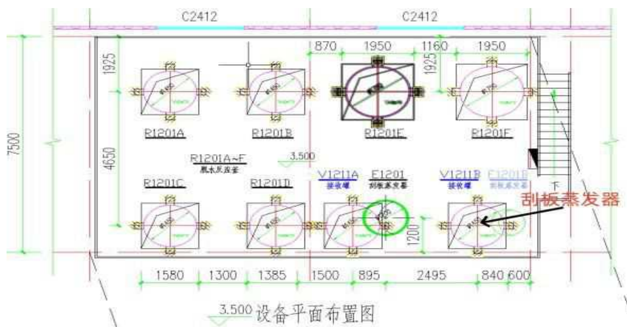
设备平面图
