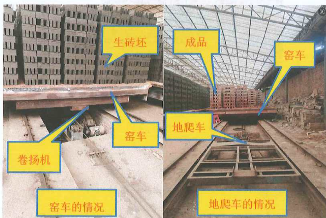
图4 窑车情况图
