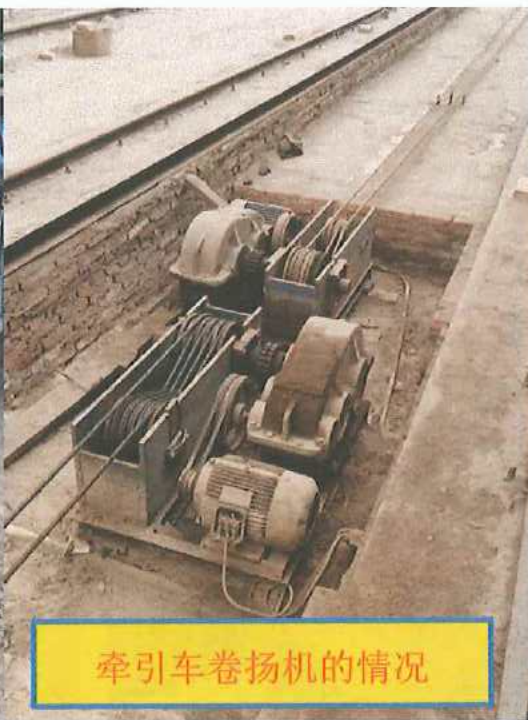
图 7 牵引车卷扬机情况图
