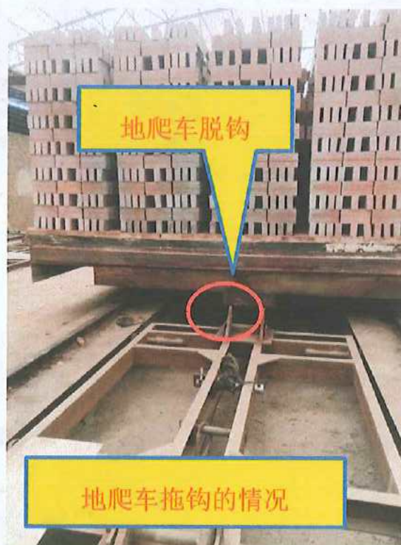
图10 地爬车拖钩情况图
