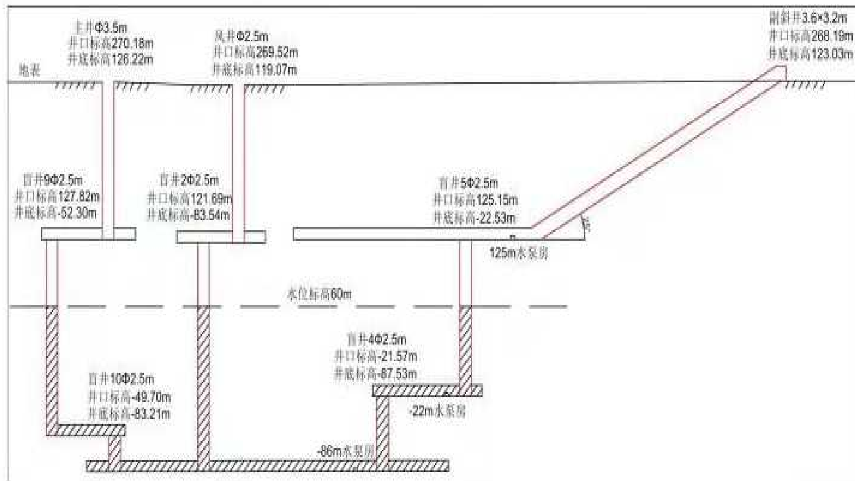
图 1 目前开拓系统纵投影示意图
