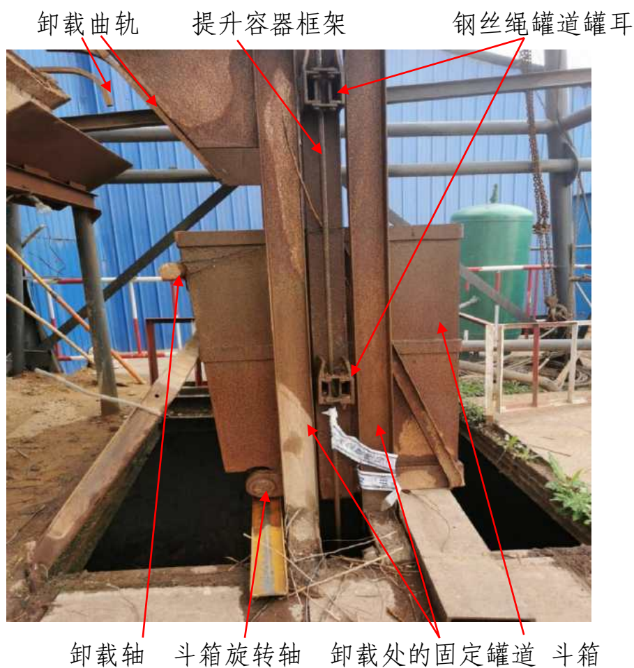
图 2 提升容器
