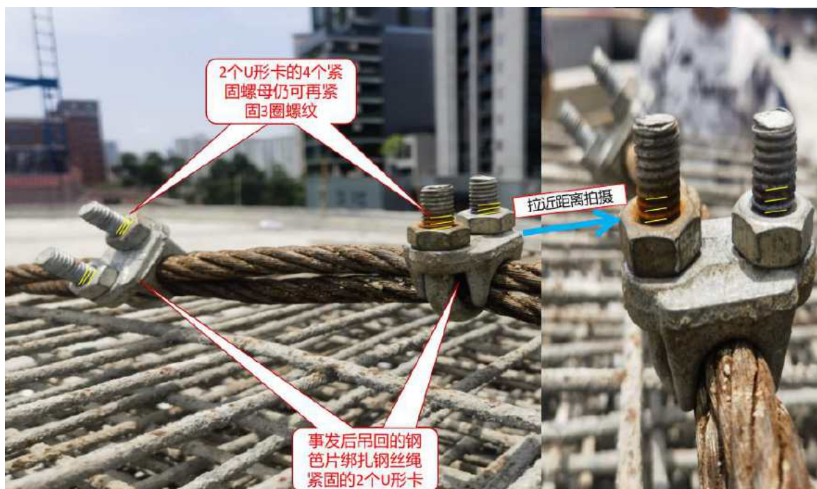
图 20 钢笆片绑扎钢丝绳 U 形卡紧固情况测试图
