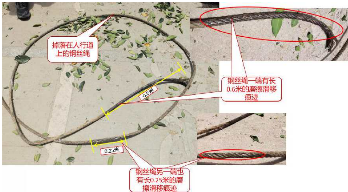
图 14 坠落在人行道上的钢丝绳勘查图
