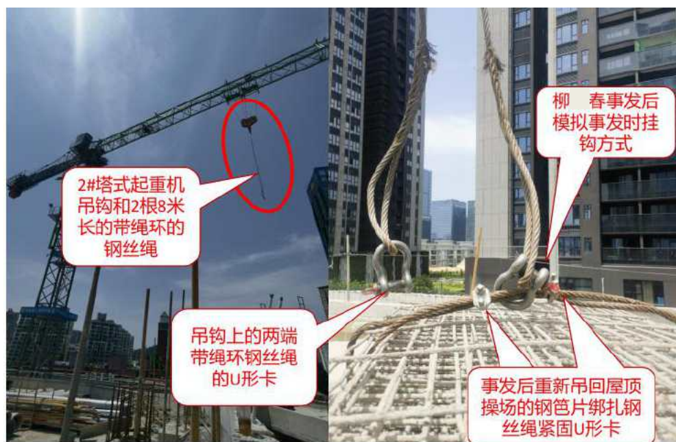
图 19 事发钢笆片吊运挂钩情况模拟图
