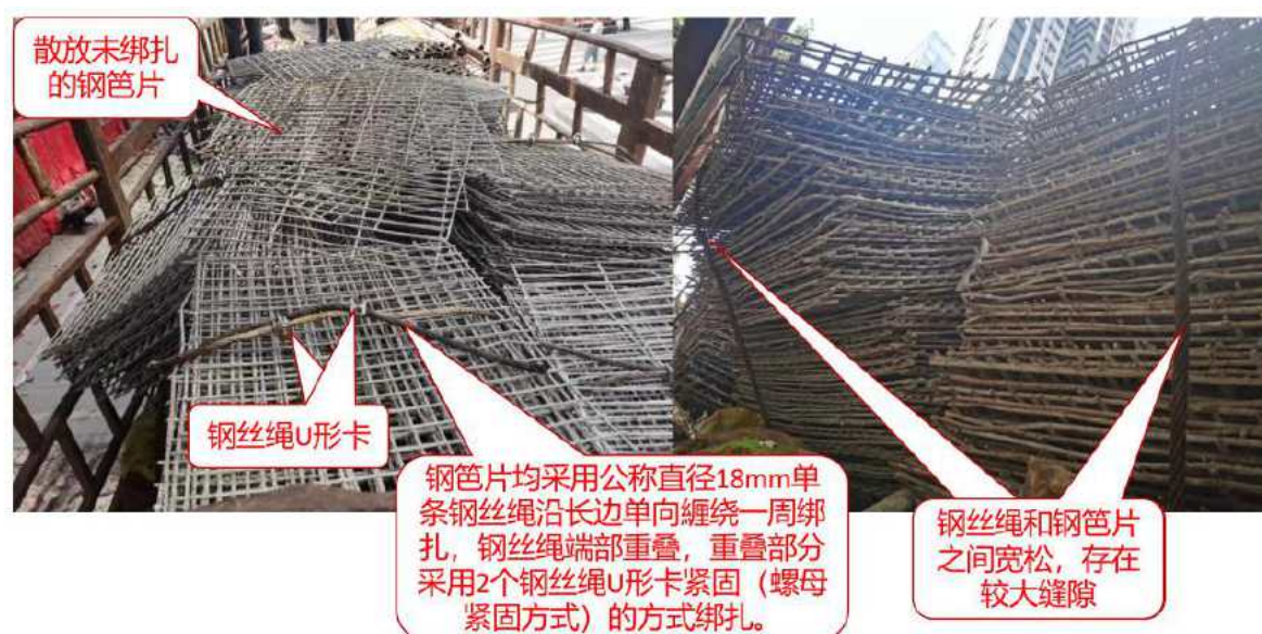
图 12 货车车厢内钢笆片勘查图
