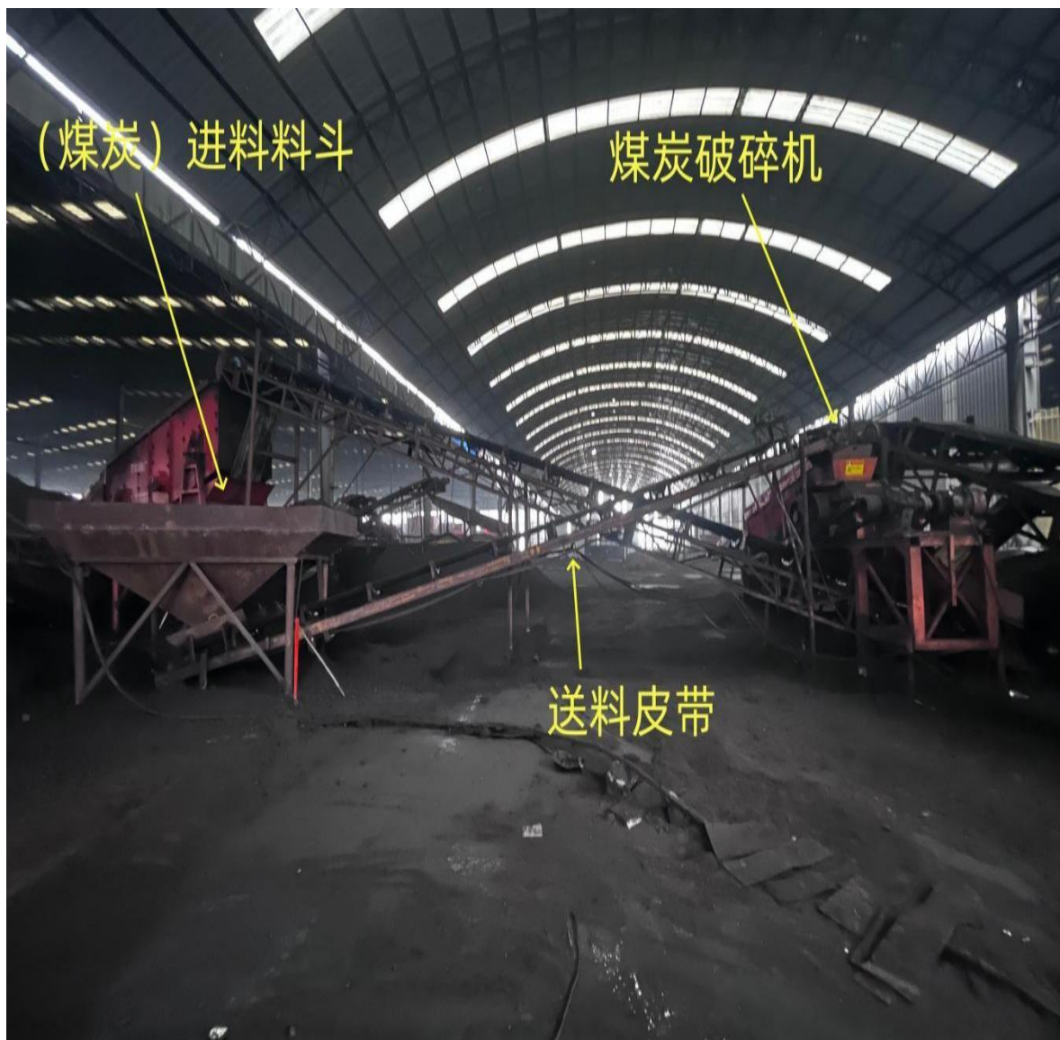
现场同类型机械图片
