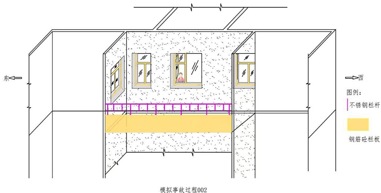
图 14 模拟事故过程 2
