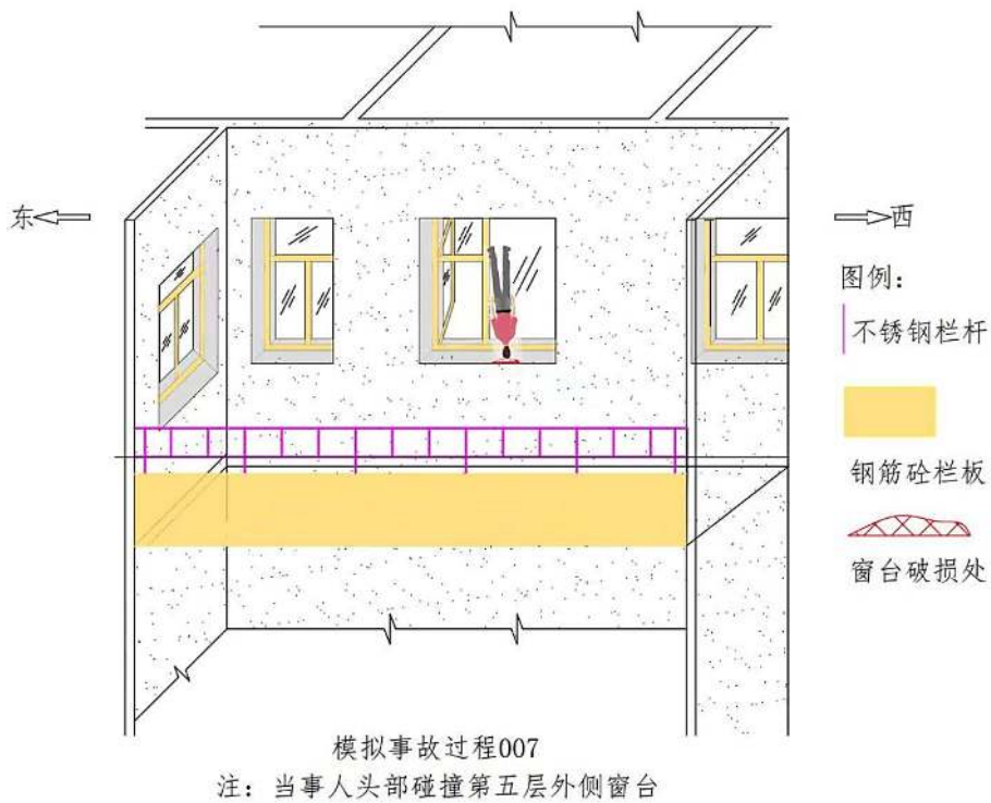
图 19 模拟事故过程 7
