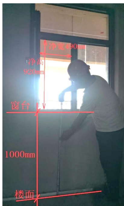
图 11 35#楼 X003 次卧窗户（西户）
