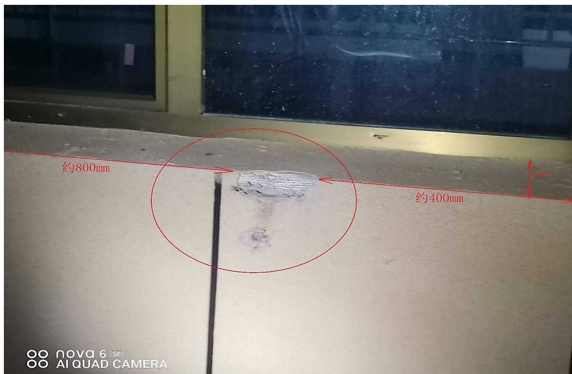
图 7 35#楼 7 层书房窗户（东户 7002）外窗台砸压痕迹
