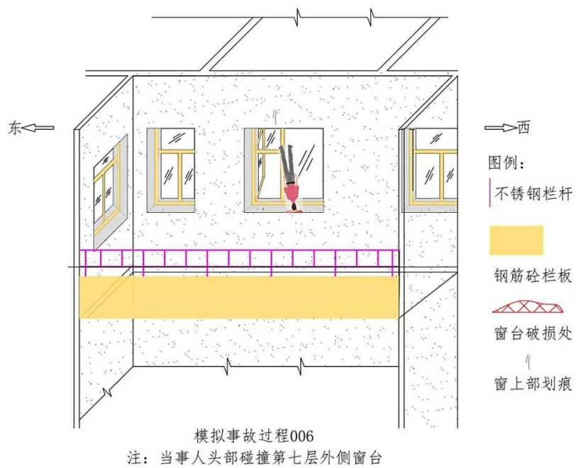
图 18 模拟事故过程 6
