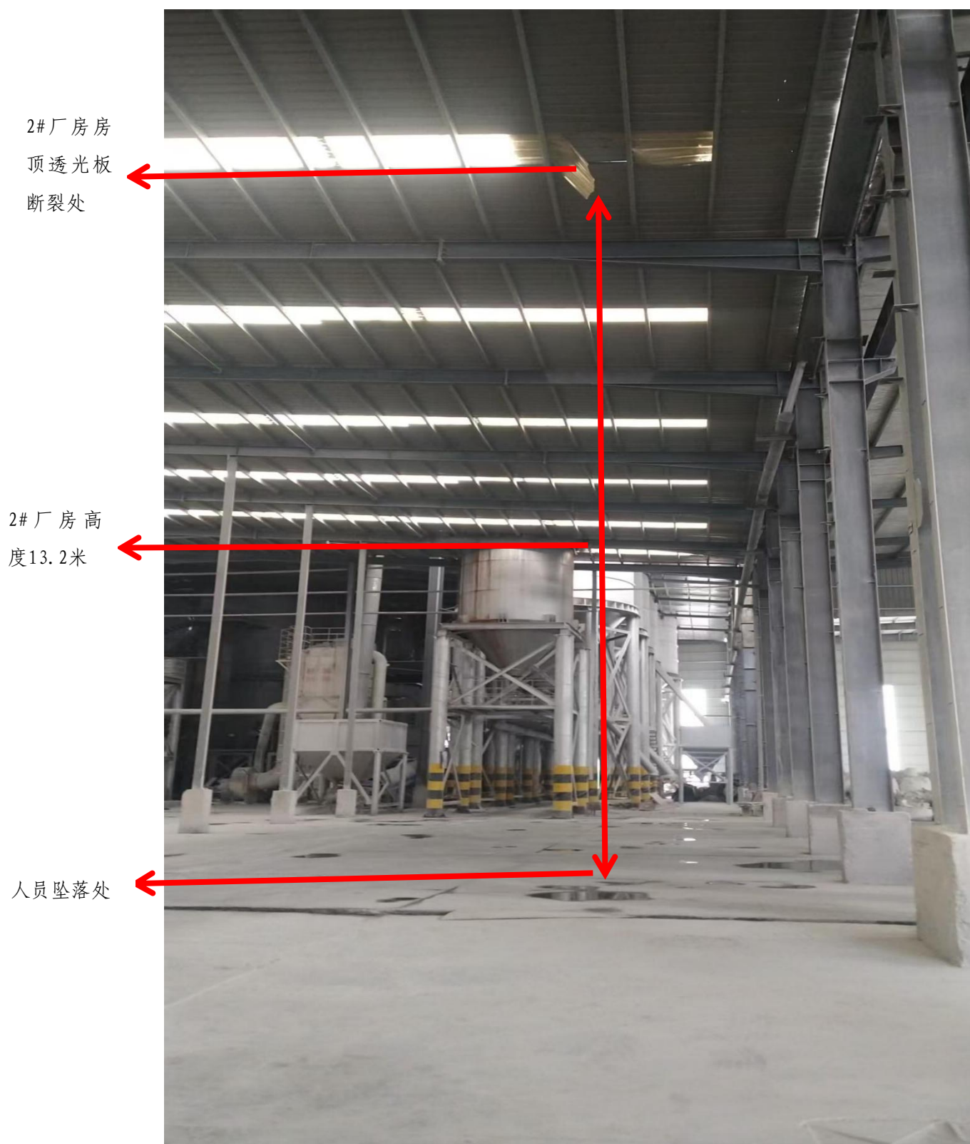
图2 事故现场图
