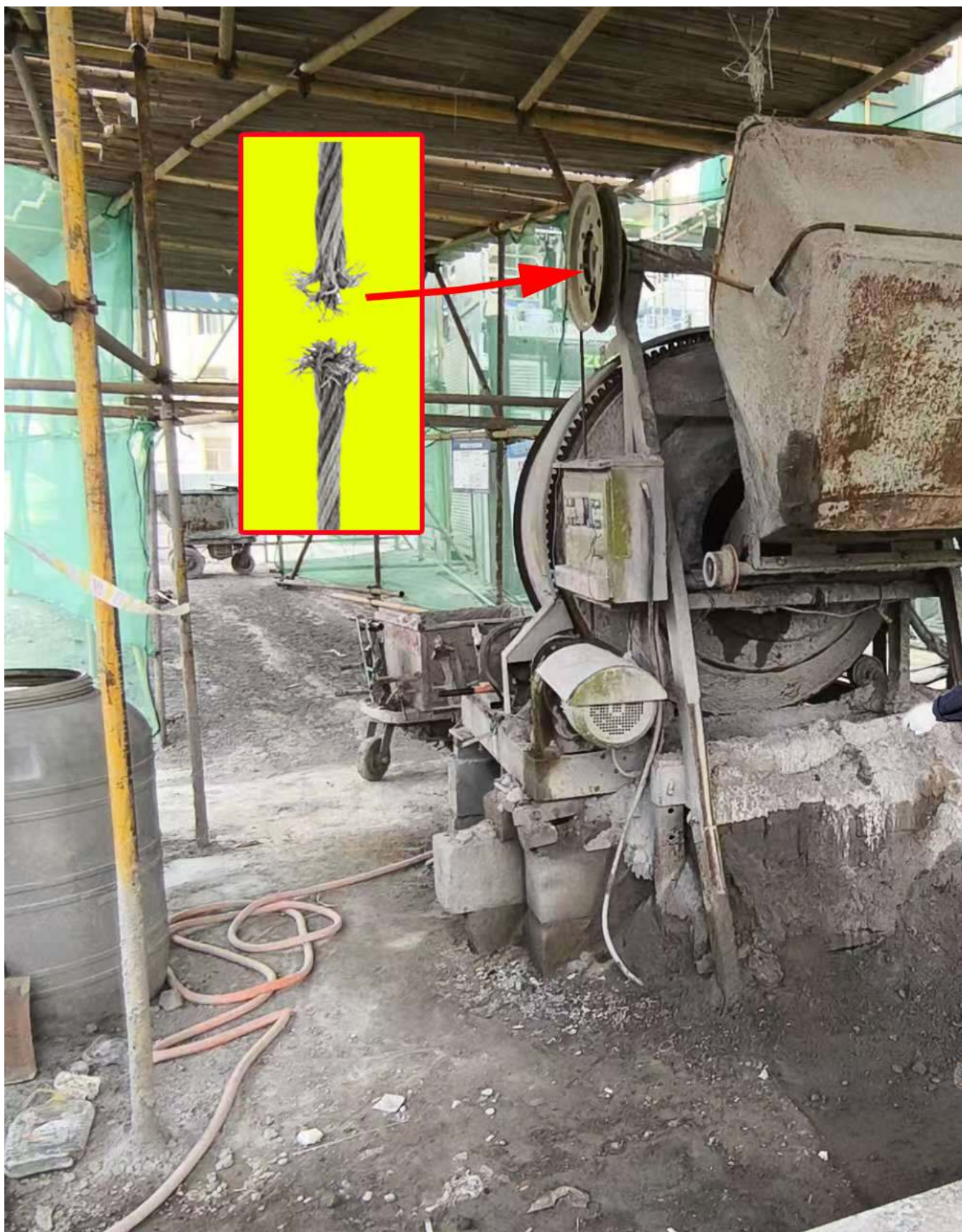
图二：事故发生时钢丝绳断裂模拟图
