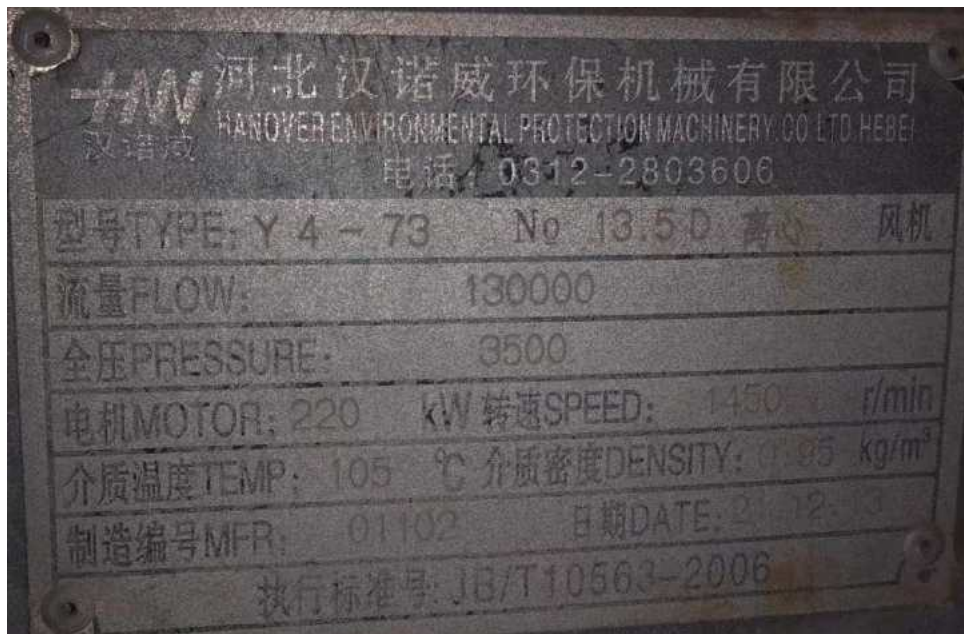
图9 1#2#钢立窑共用的引风机铭牌
