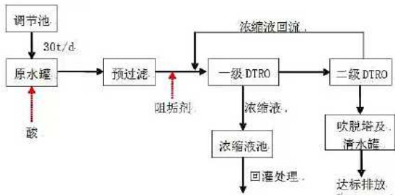
两级DTRO工艺流程图
