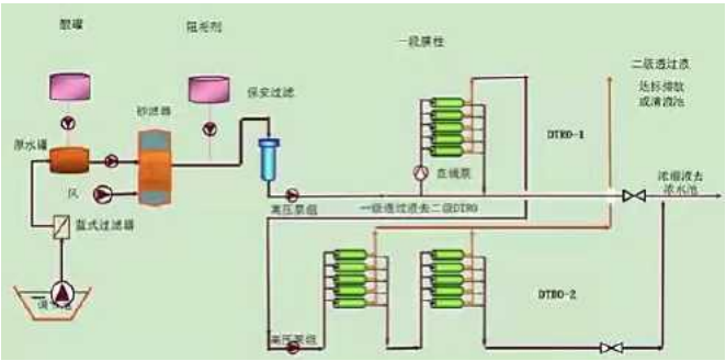
两级DTRO工艺流程图
