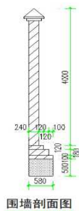
图 2 实际施工图纸
