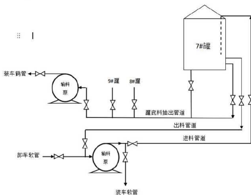
图 2 7 号罐相关工艺流程简图
