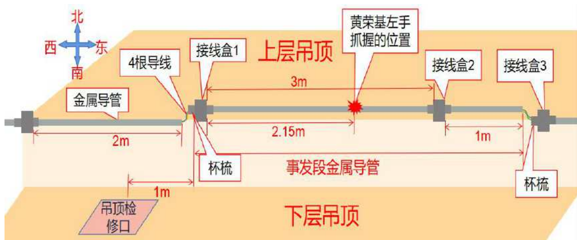
图 13 事发金属导管连接状态和黄荣基手抓握位置图
