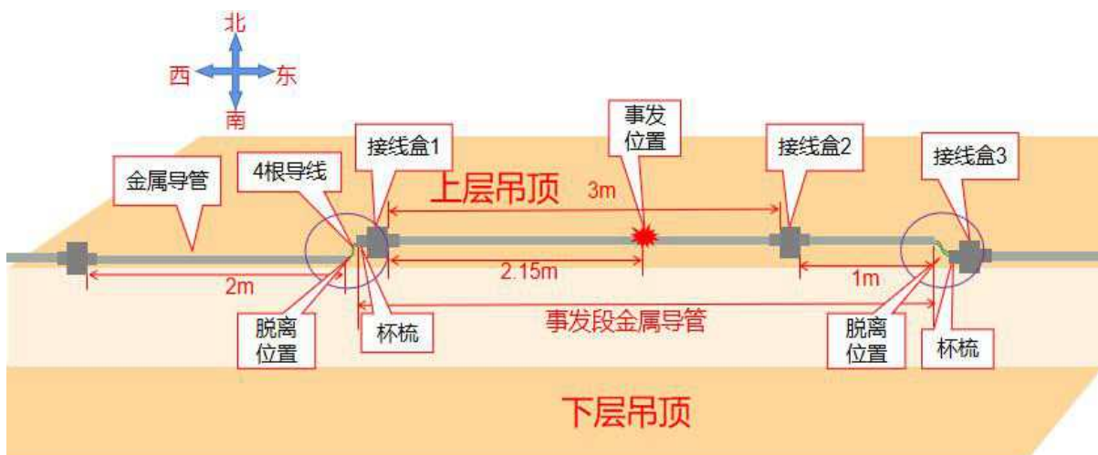
图 31 事发段金属导管丧失电气连续性示意图
