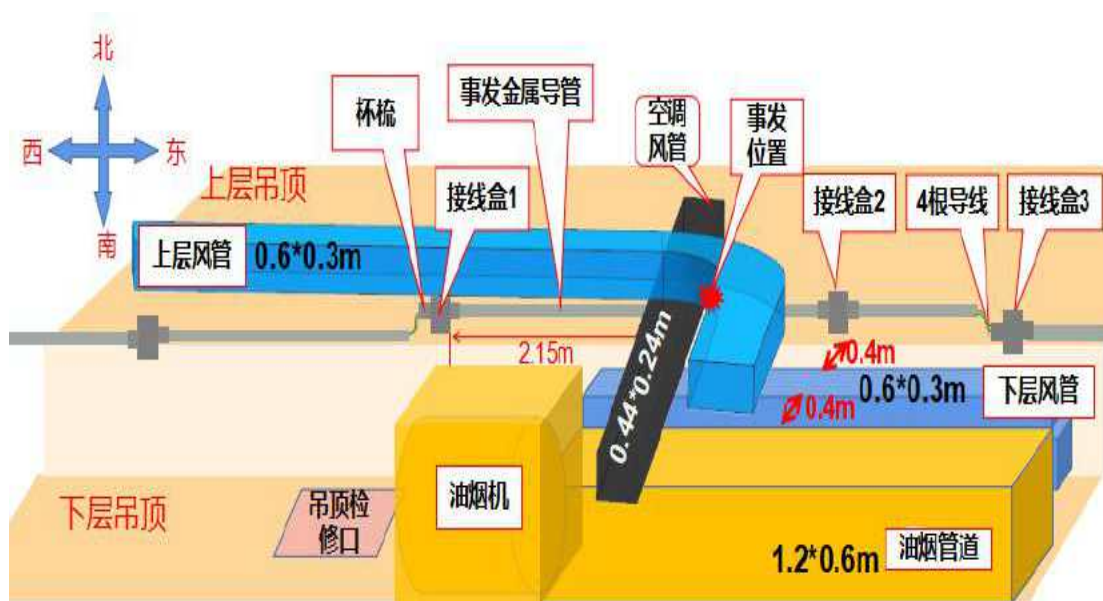
图 6 事发吊顶内设备、管道布置图
