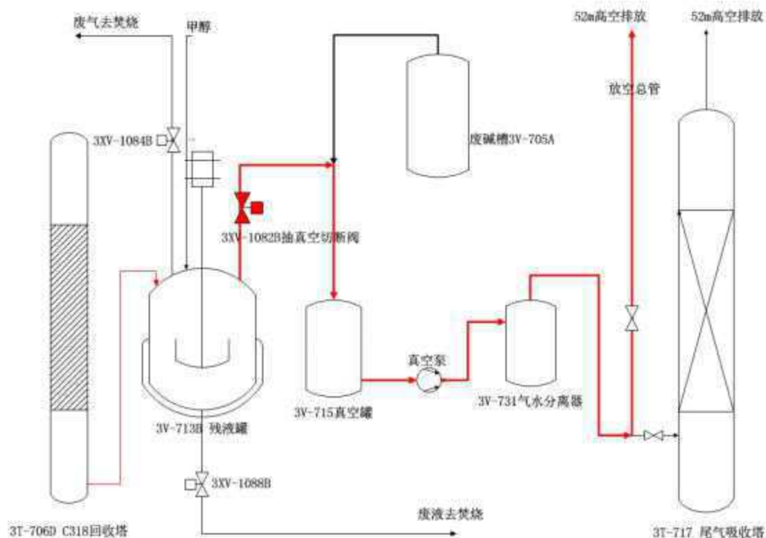
有毒气体排放路径示意图
