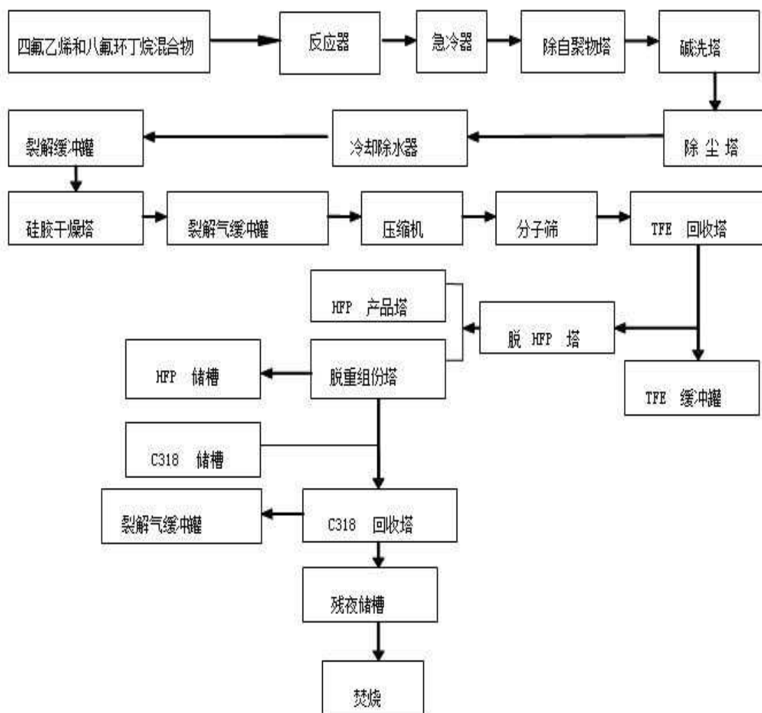
3HFP 装置生产工艺流程图
