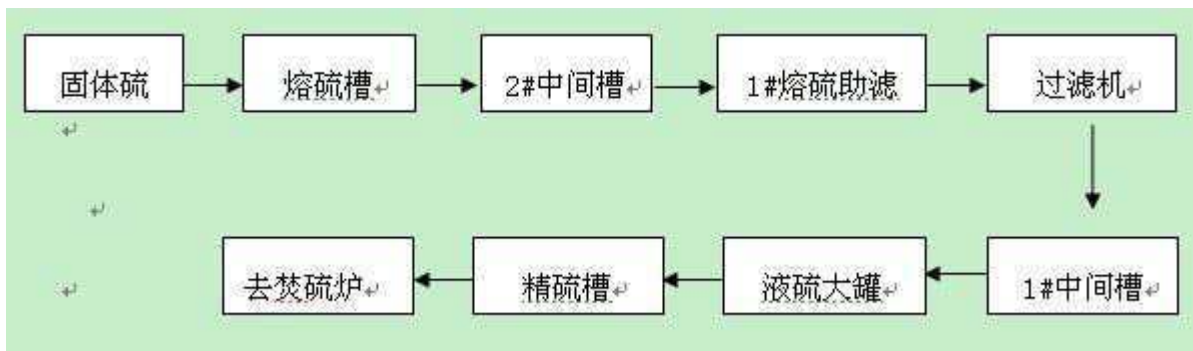
熔硫工艺简图
