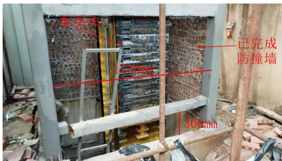
图 7 事故现场勘查图（自西往东）
