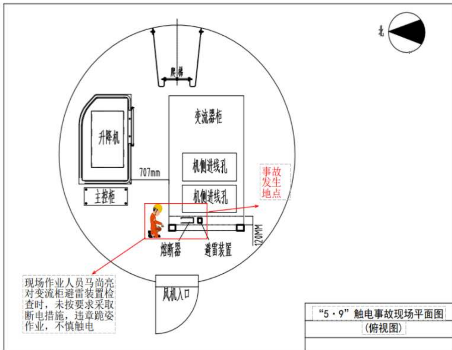
图 1·· “5·9” 事故现场平面图（俯视图）
