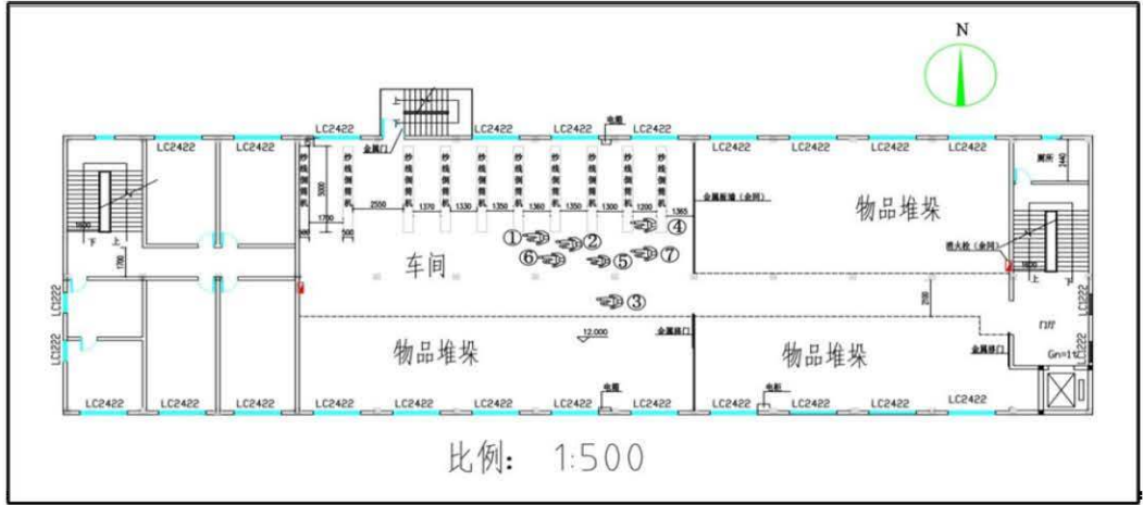
图 4 库房四层平面图
