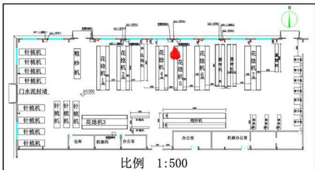
图 2 花捻车间平面布置图
