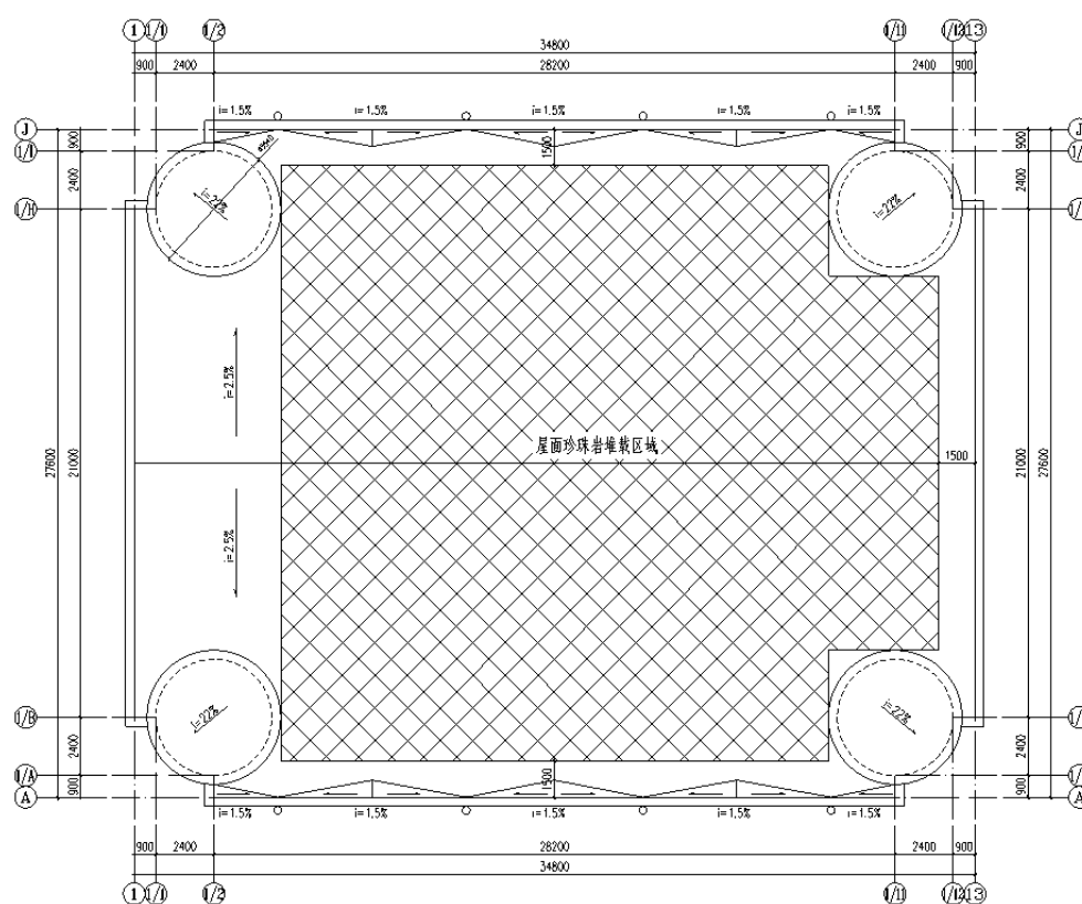
图3 屋面堆载珍珠岩范围示意图
