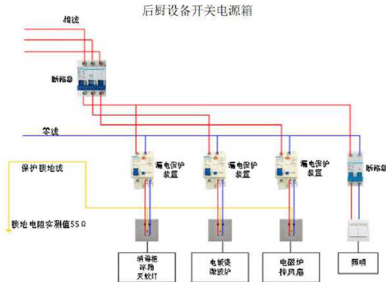
图 20 后厨设备开关电源箱线路及电气示意图
