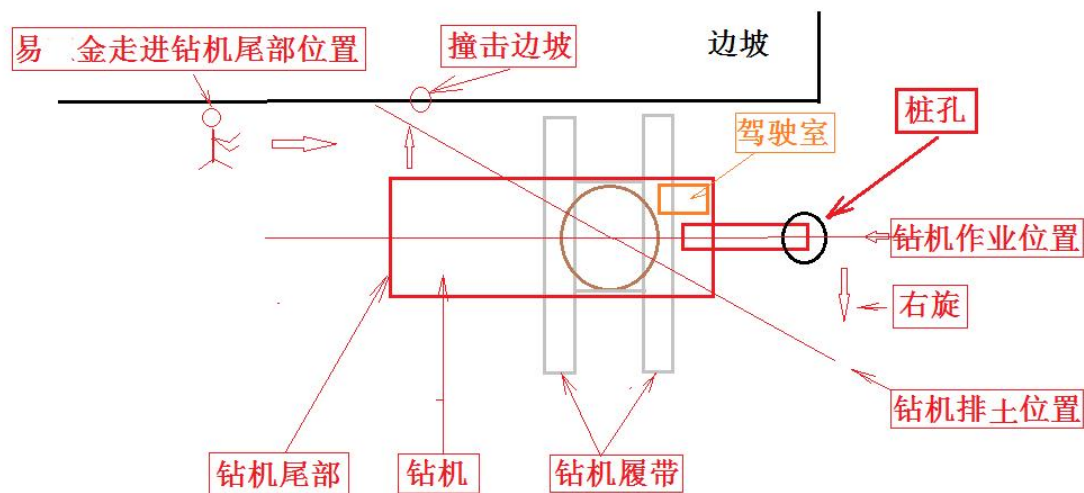
钻机正常作业及排土作业的示意图
