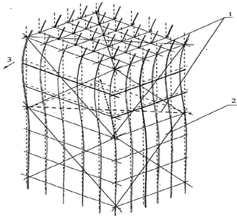
图 8 满堂支撑架整体失稳 1—水平剪刀撑；2—竖向剪刀撑；3—失稳方向
