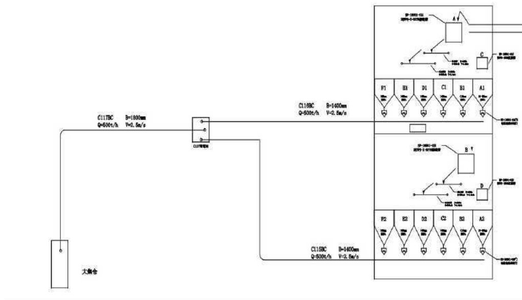
工艺流程图
