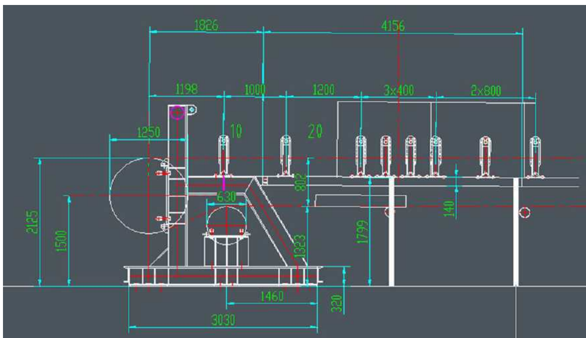
管状带式输送机机尾安装图
