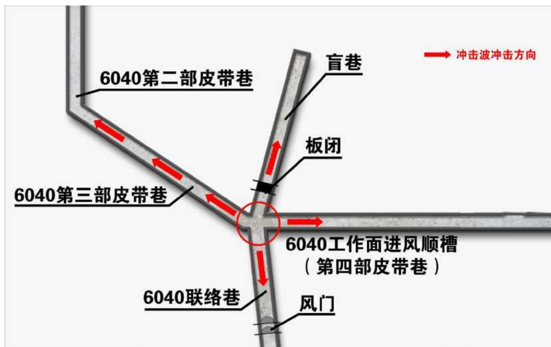
图 7 盲巷口爆炸冲击波方向示意图
