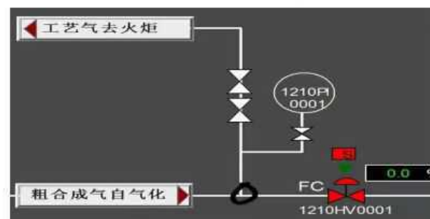
图7 主管线与放空火炬管线连接处堵塞图
