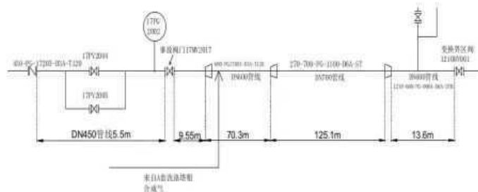
图9 止回阀与界区阀之间管道（管道长 224.05m）
