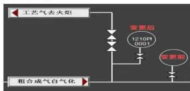
图6 远传压力变送器变更图
