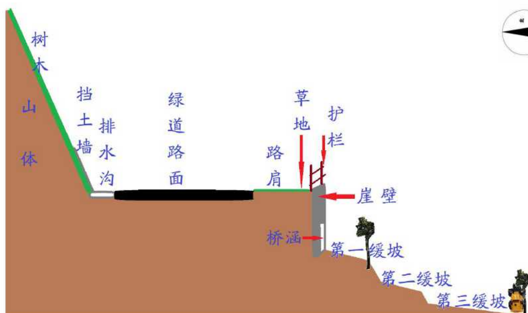
图5 事发位置剖面图
