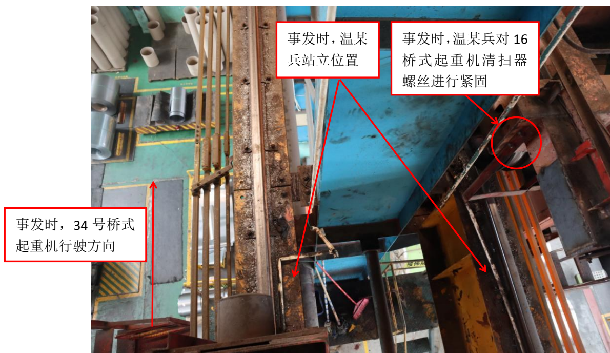
图 2 事故现场情况
