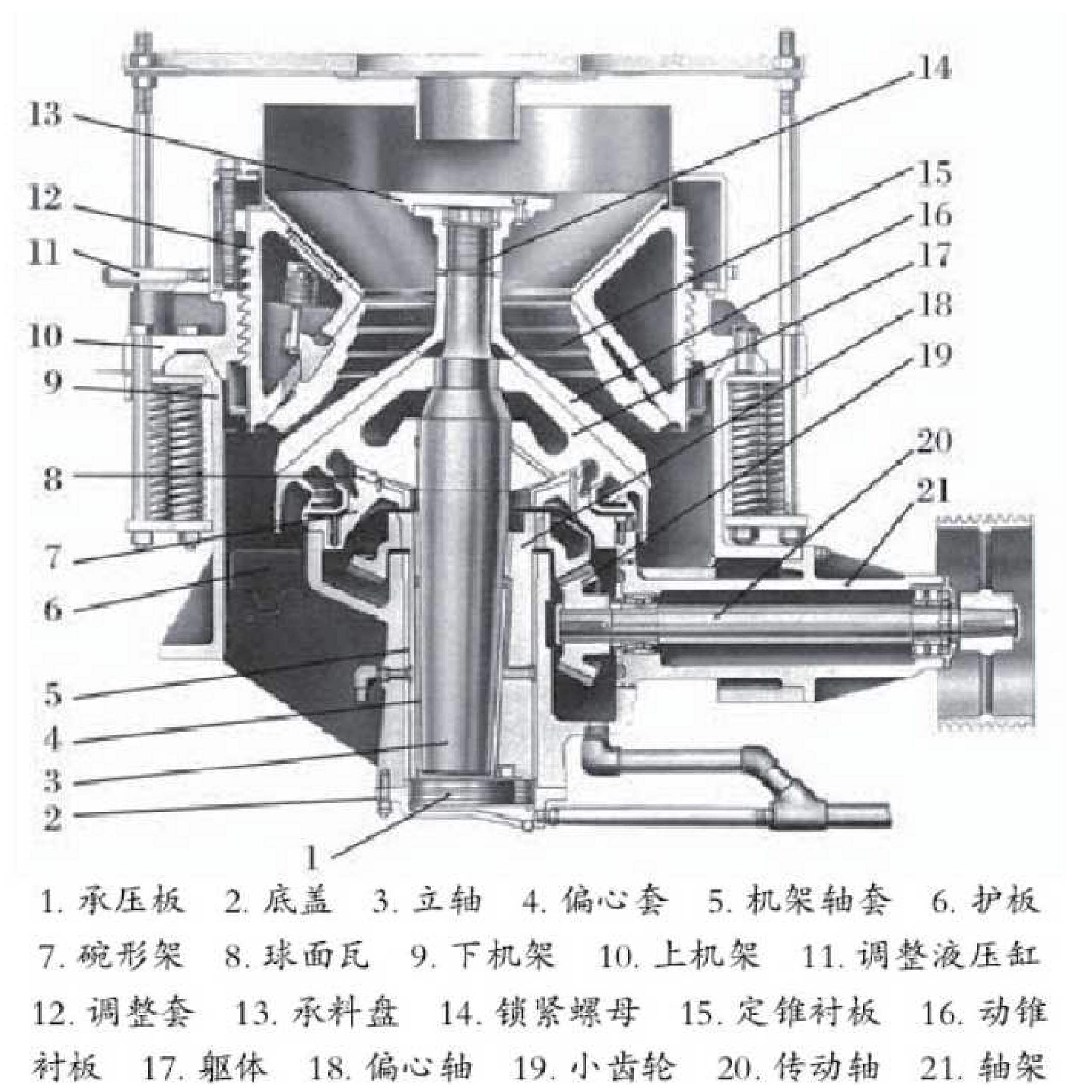
图 6 圆锥破碎机内部构造图
