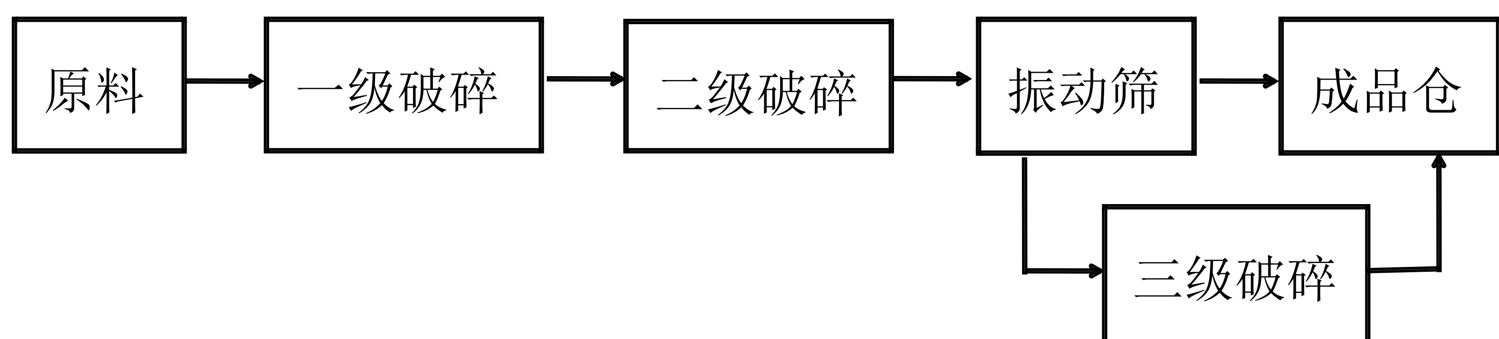
图 4 1060 破碎线工艺方框图
