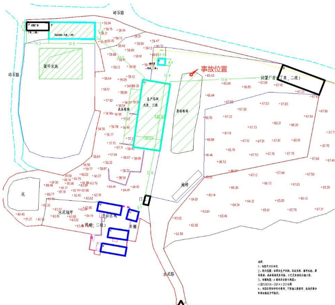
(该图为云鼎建材公司平面布置图)
