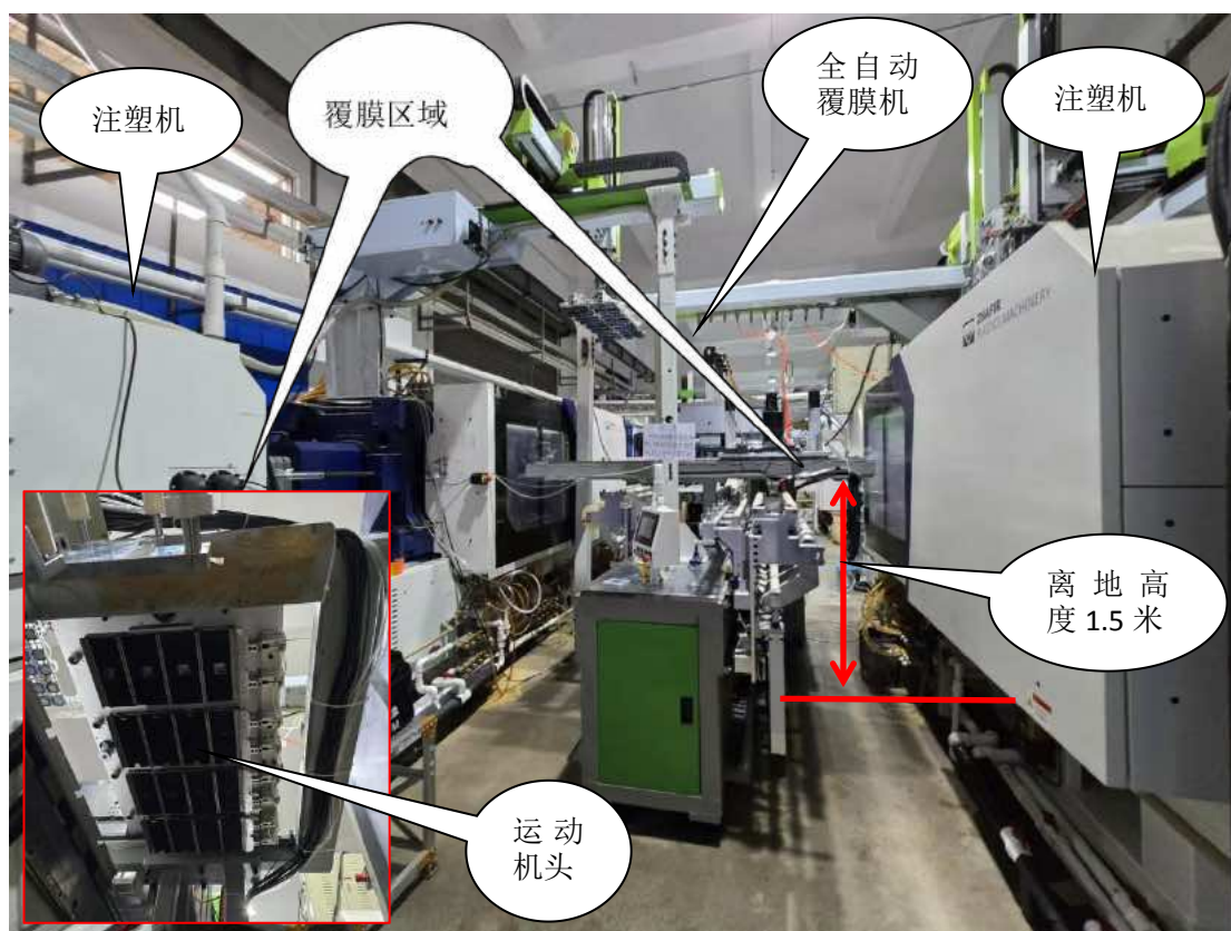
图1 涉事自动化机械设备 90B7 号线
