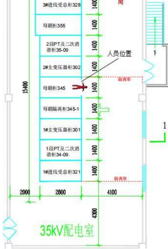
35KV 配电室平面图
