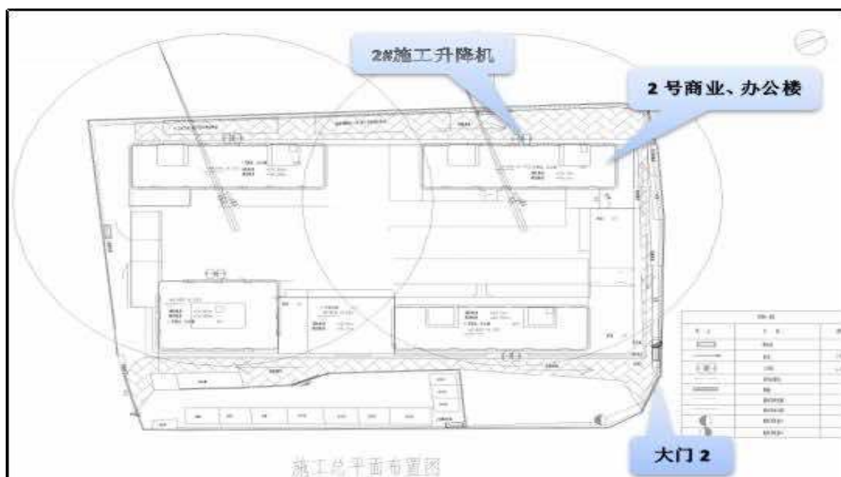
图 1 施工总平面图
