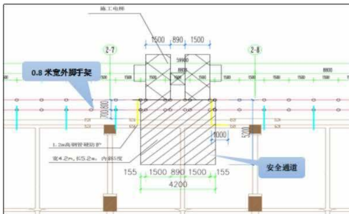
图 6 18 层楼层门及安全通道示意图二
