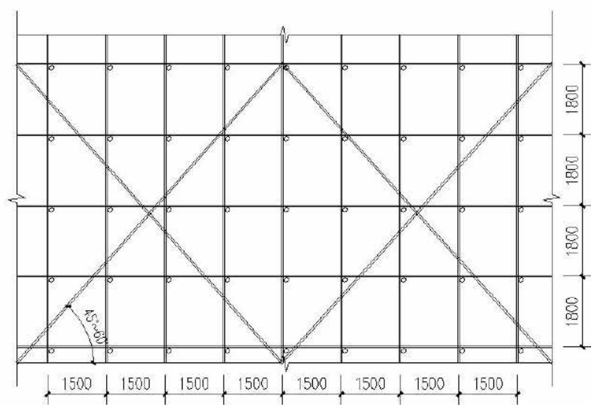
落地式钢管脚手架立面图
