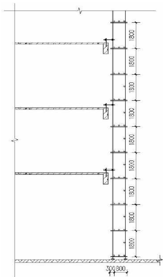
图 4 落地式钢管脚手架剖面图
