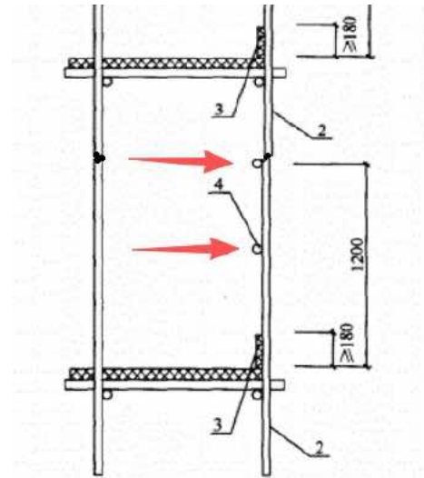
图 7.3.12 栏杆与挡脚板构造 1—上栏杆；2—外立杆；3—挡脚板；4—中栏杆
