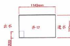
粪污管道检修口俯视图
