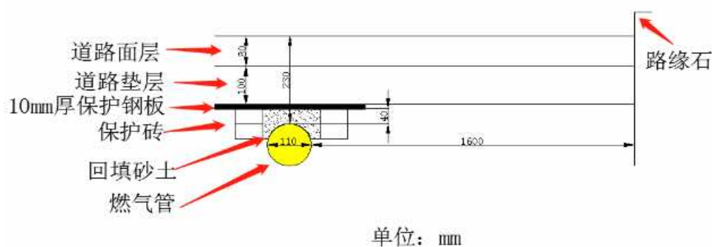
图2 横断面图
