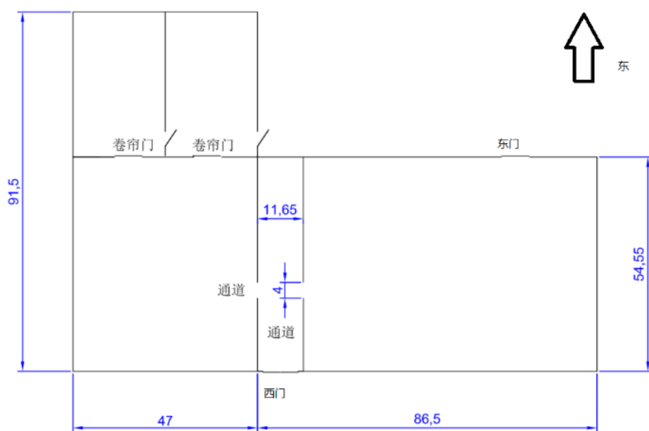
图 9 厂房建筑结构
