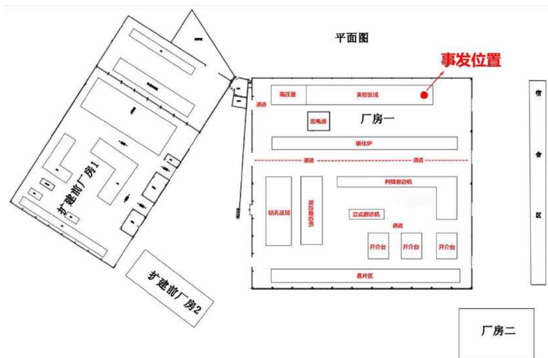
图1 厂房平面图
