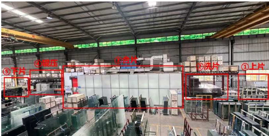
图2 干夹线现场图
