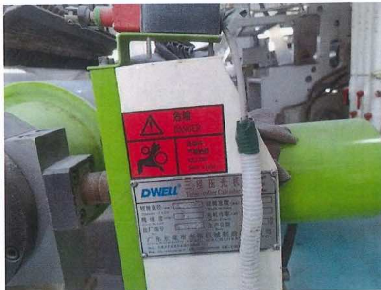
图2 涉事三辊压光机标牌（李建红提供，拍摄时间：2021年7月11日）
