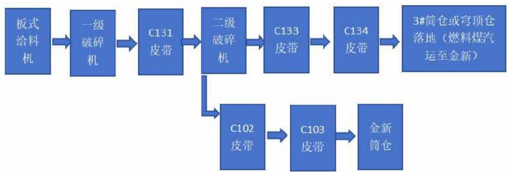
图 1 工艺流程图
