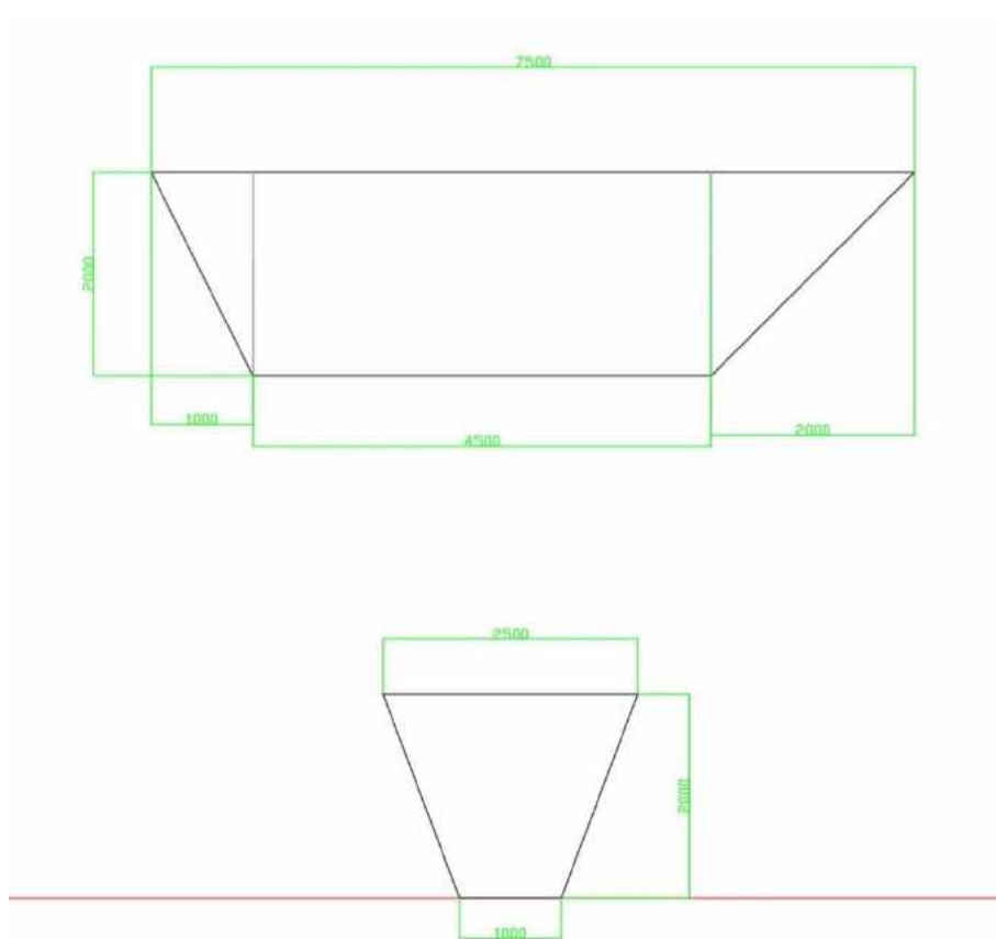
图 1：简易水箱形状图纸
